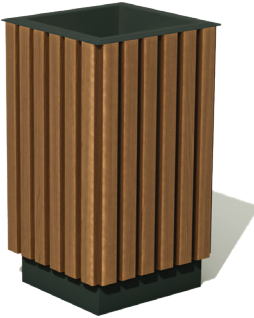
Урна UR 106 ☑ Арт. 30106 📏 350 x 350 x 600
