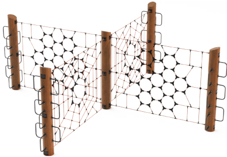
Спортивный элемент SC 112 ✓ Арт. 23112 ▮ 8900 x 8900 x 3000 ⚡ 11900 x 11900
