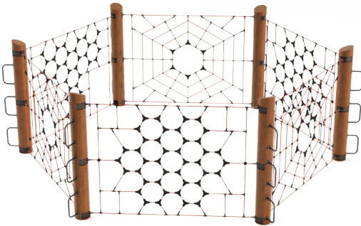
Спортивный элемент SC 116 ✓ Арт. 23116 ▮ 8900 x 7680 x 3000 ⚡ 11900 x 10680
