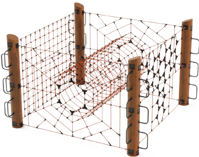
Спортивный элемент SC 109 ✓ Арт. 23109 ▮ 4900 x 4900 x 3000 ⚡ 7900 x 7900
