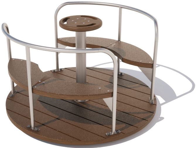
Карусель RD 104 ☑ Арт. 13104 📏 1500 x 1500 x 900 📏 5500 x 5500 👤 3-10
